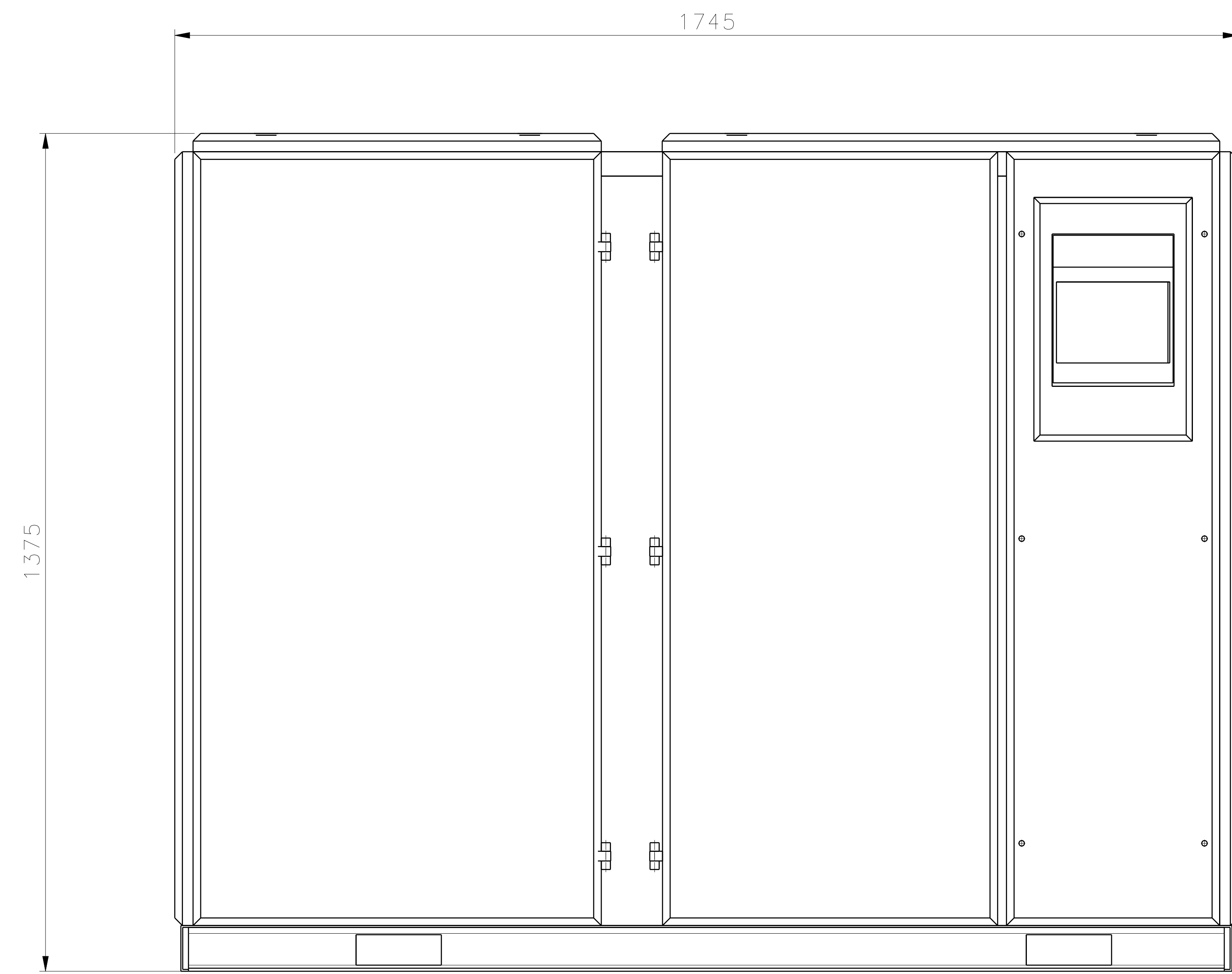
Front view Scale: 1:5
