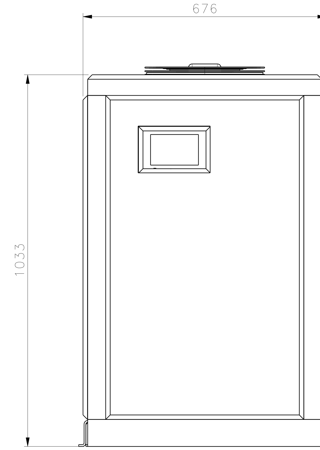
Left view Scale: 1:5
