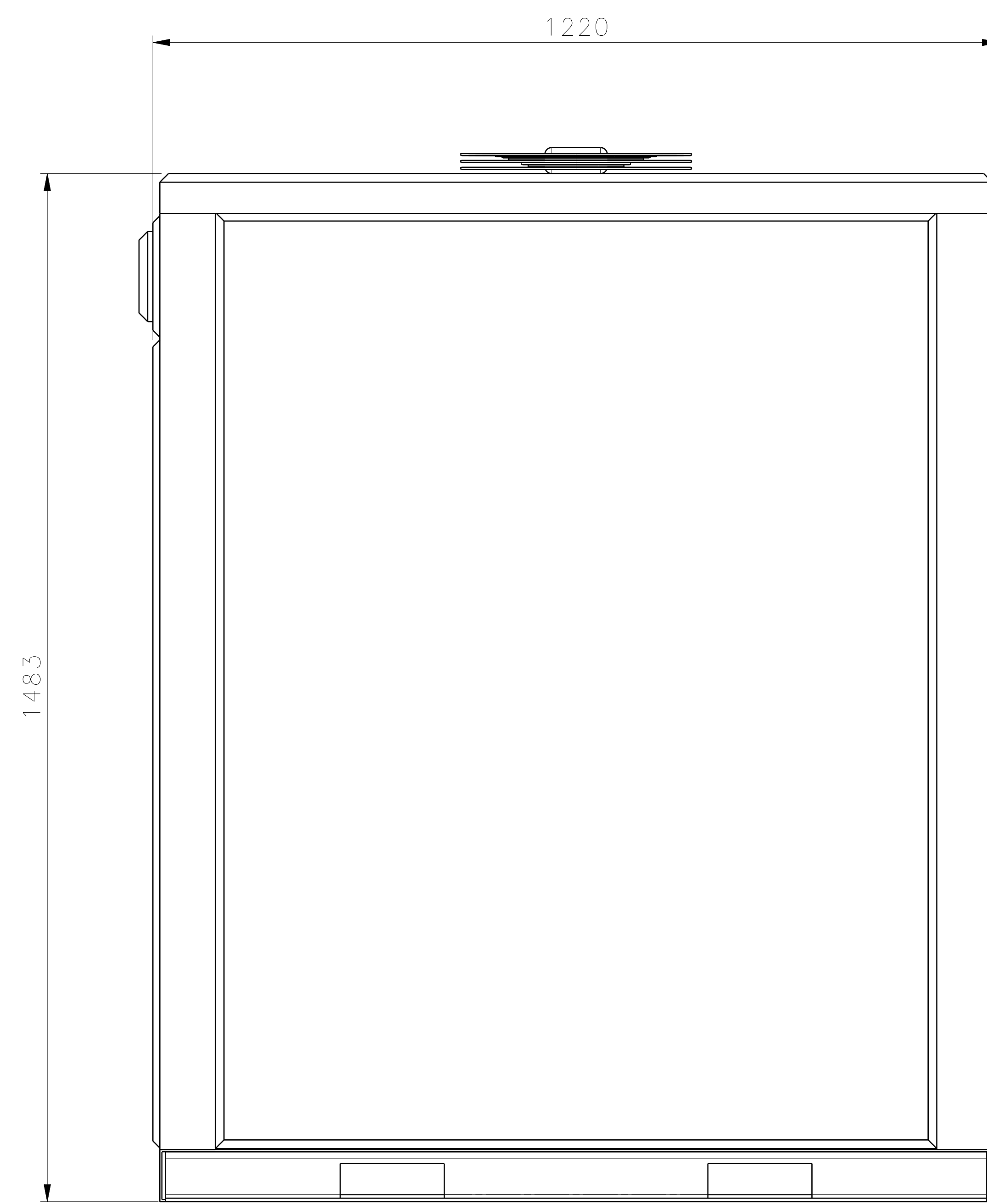
Front view Scale: 1:5
