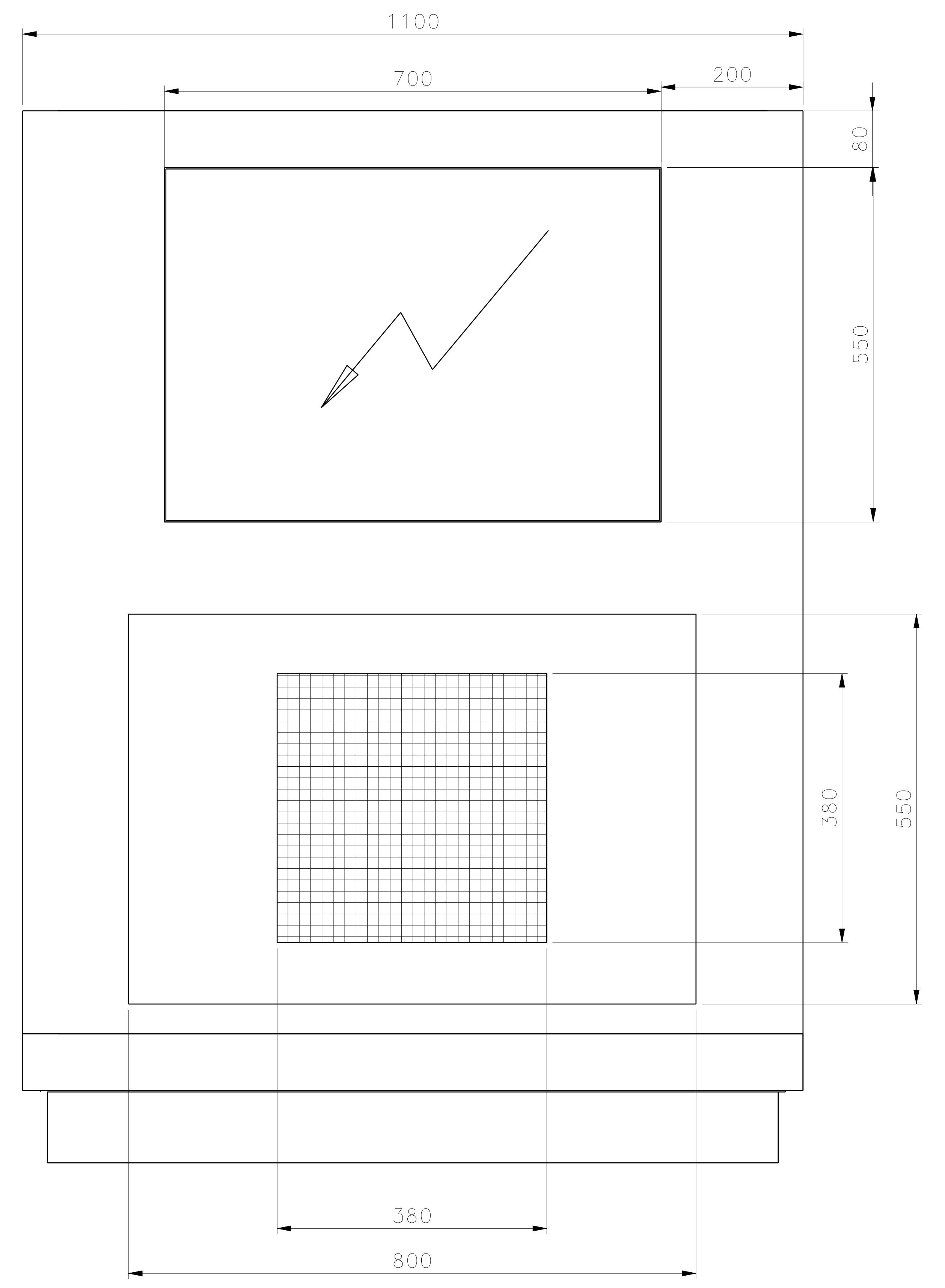
Left view Scale: 1:4
