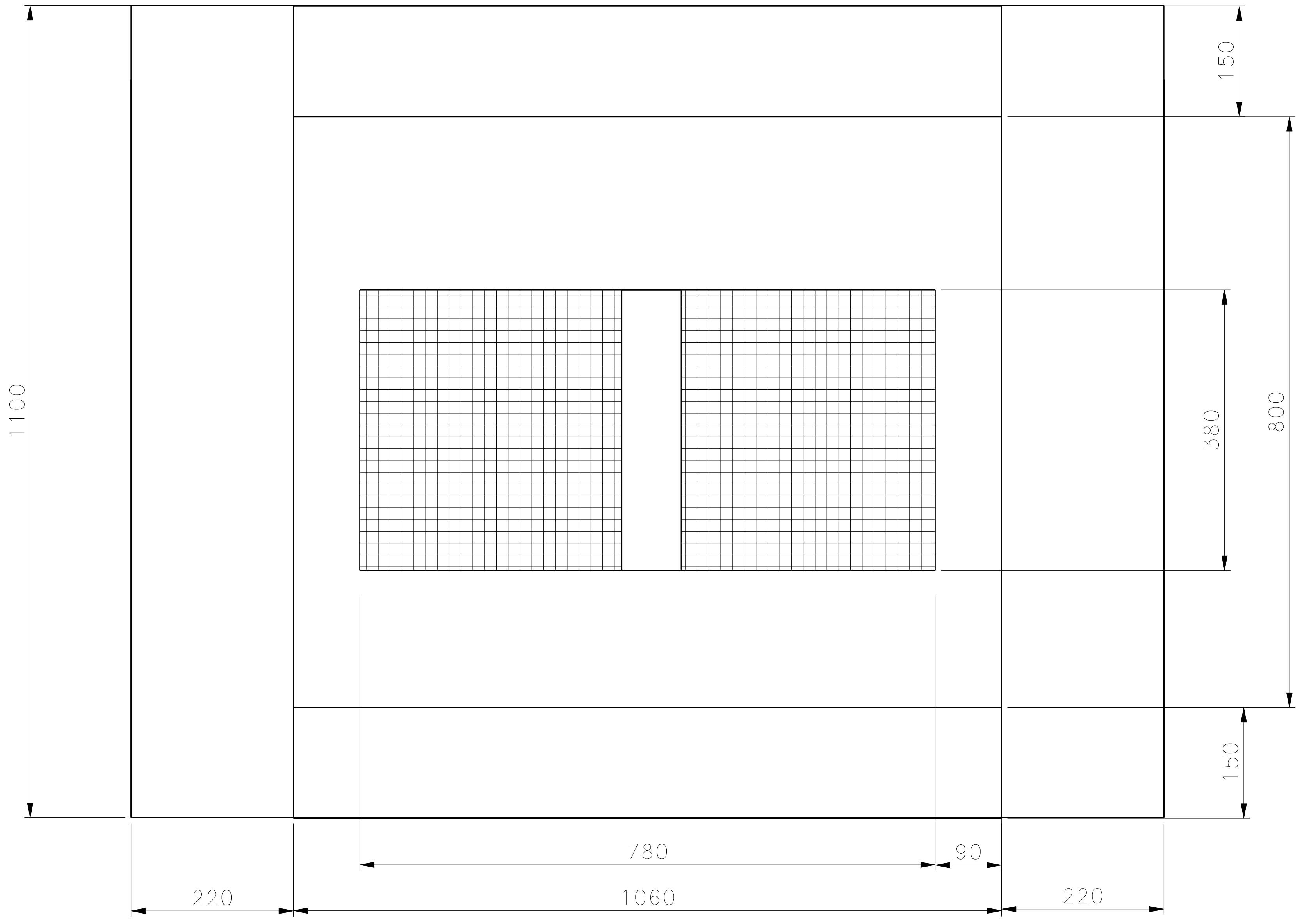
Top view Scale: 1:4
