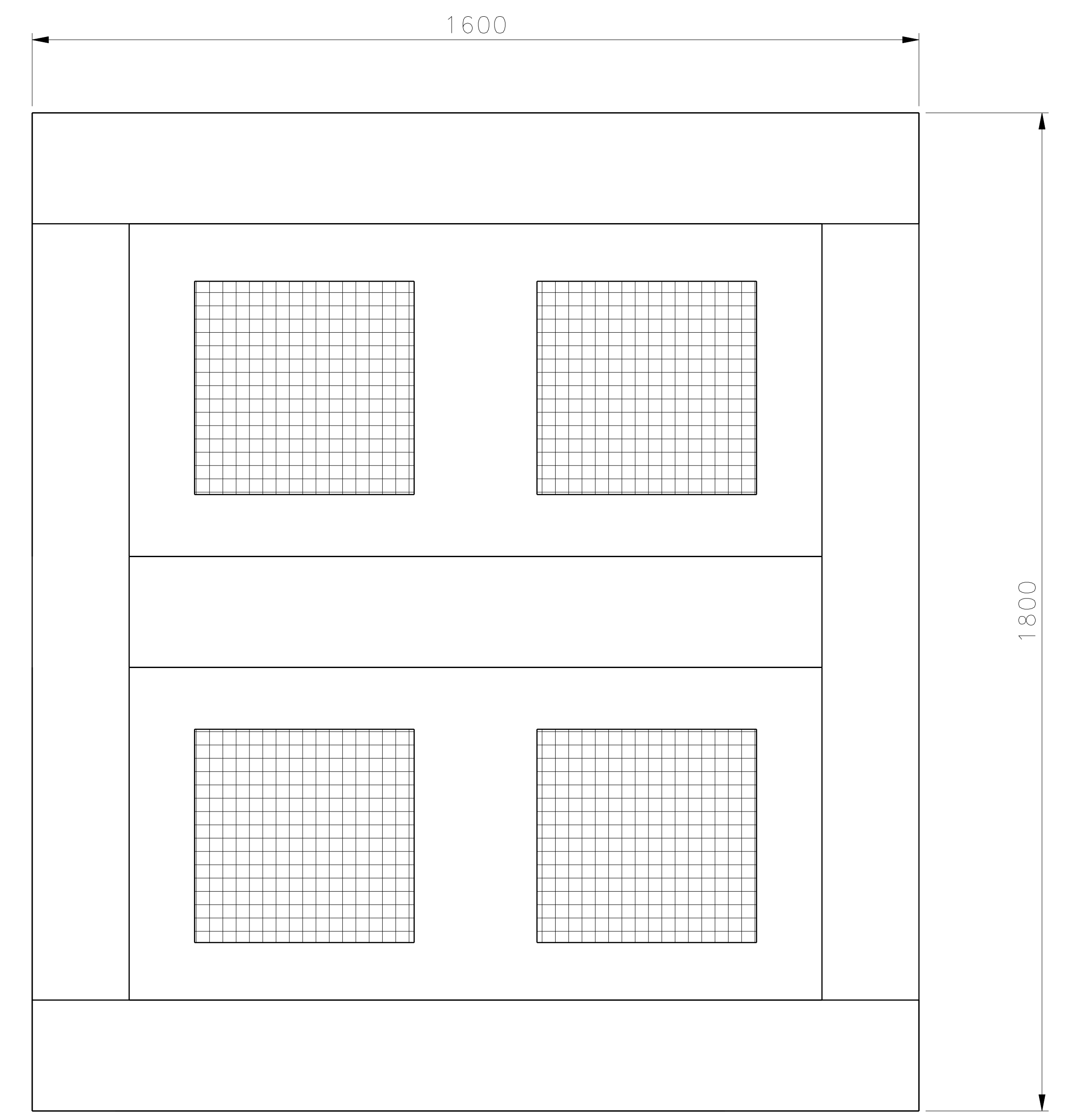
TOP VIEW Scale: 1:6
