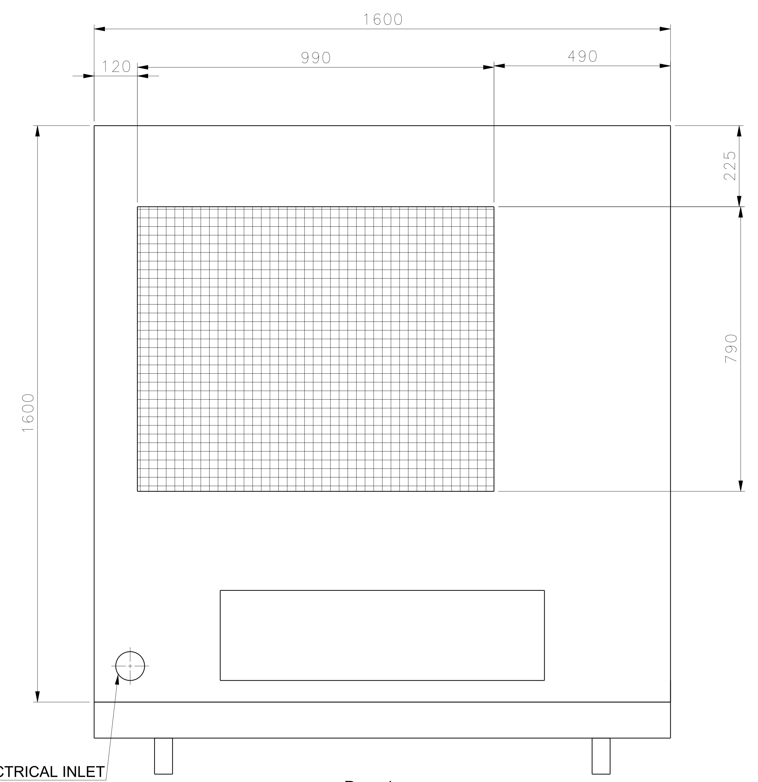
Rear view Scale: 1:6
