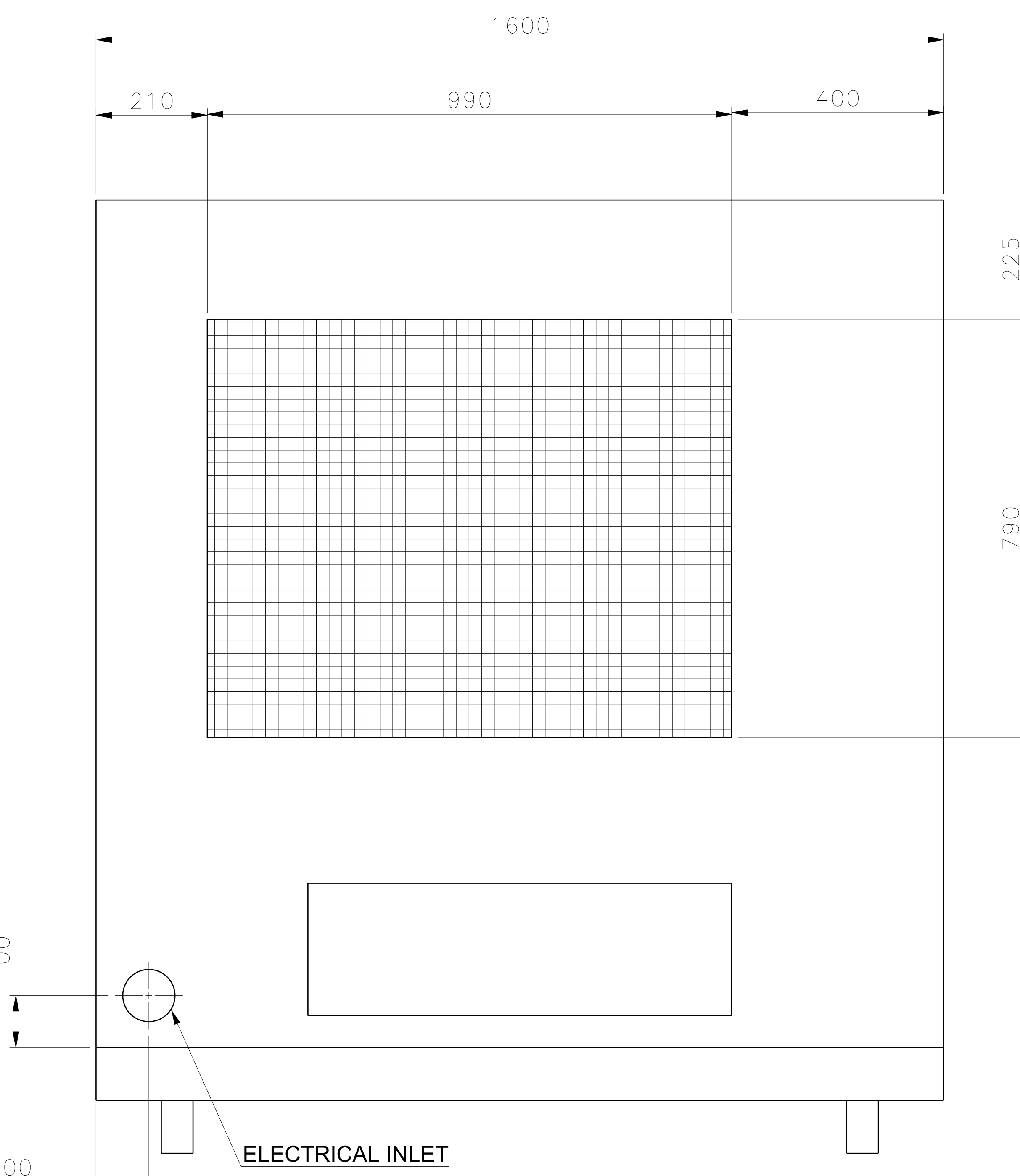
Rear view Scale: 1:6
