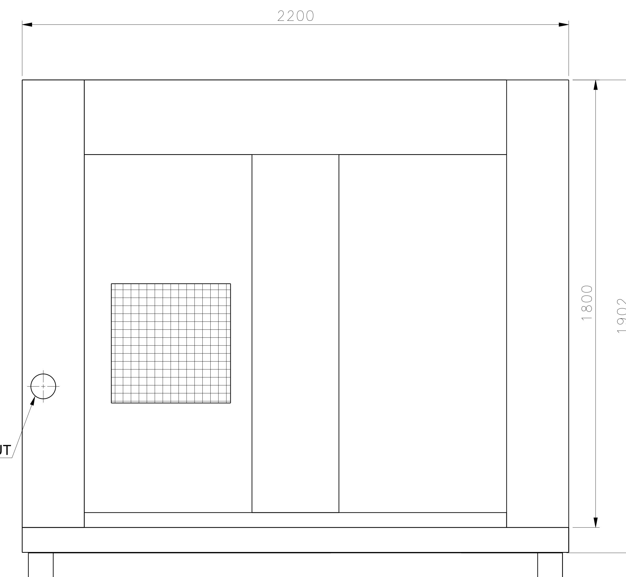
Left view Scale: 1:8
