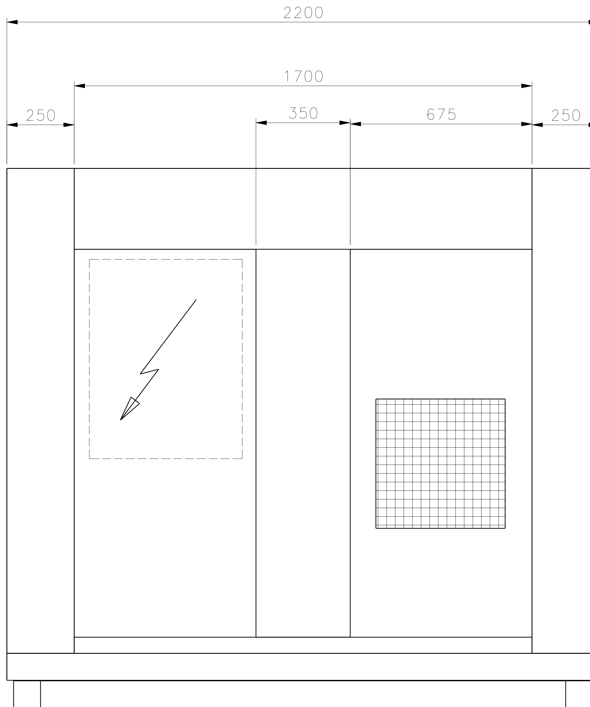
Right view Scale: 1:8
