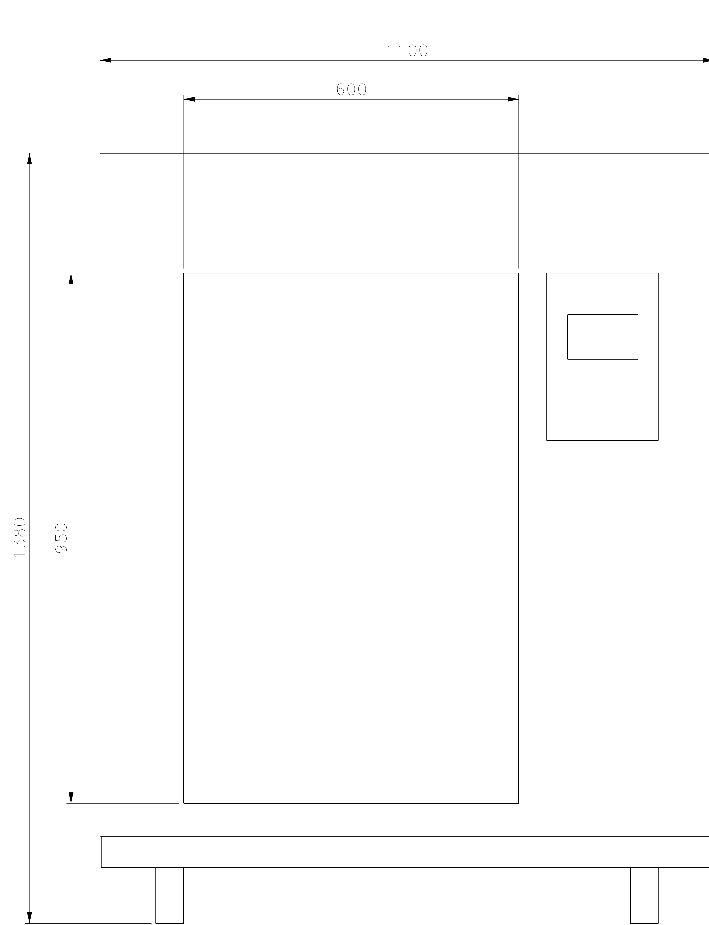
Front view Scale: 1:4
