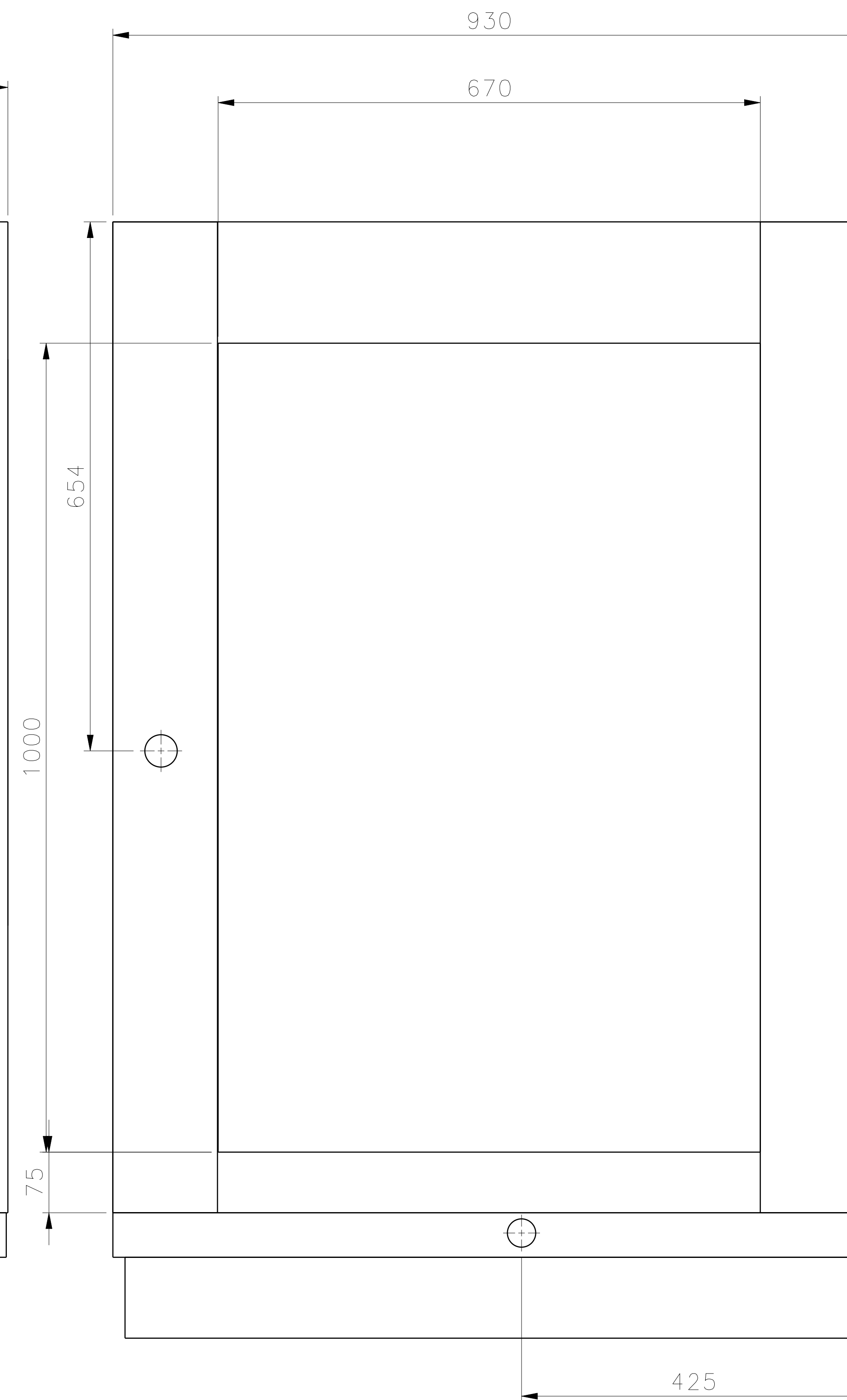
Left view Scale: 1:4
