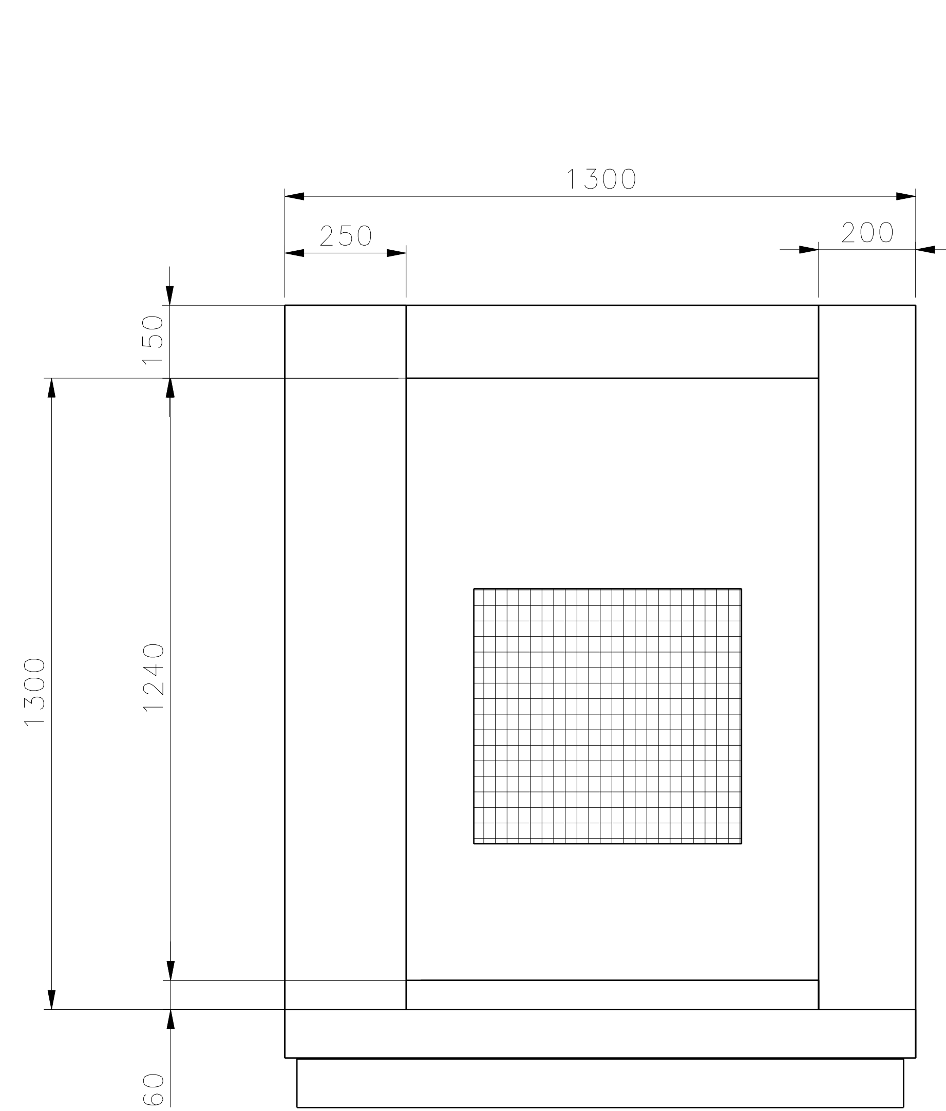
Right view Scale: 1:8
