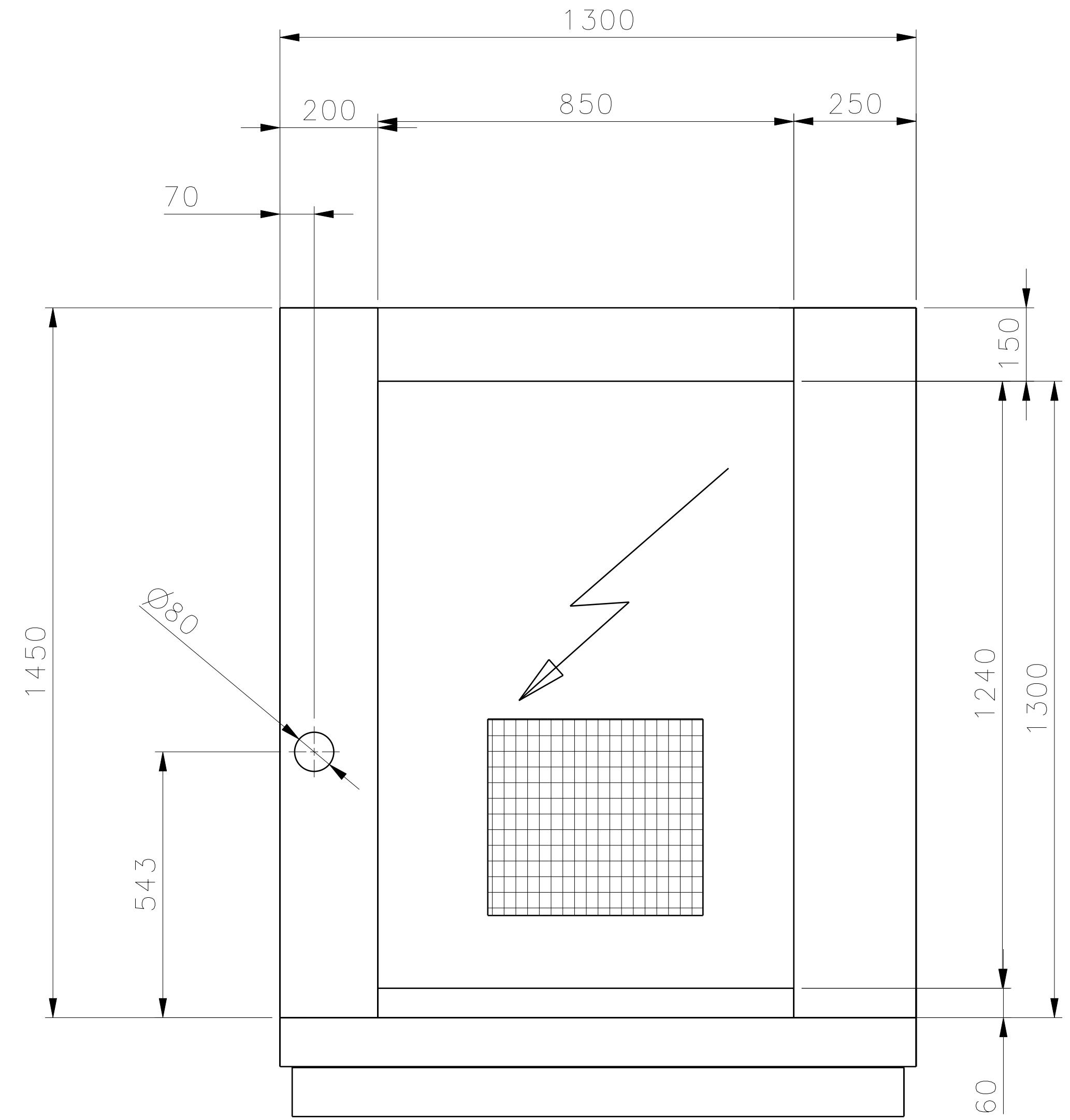
Left view Scale: 1:8
