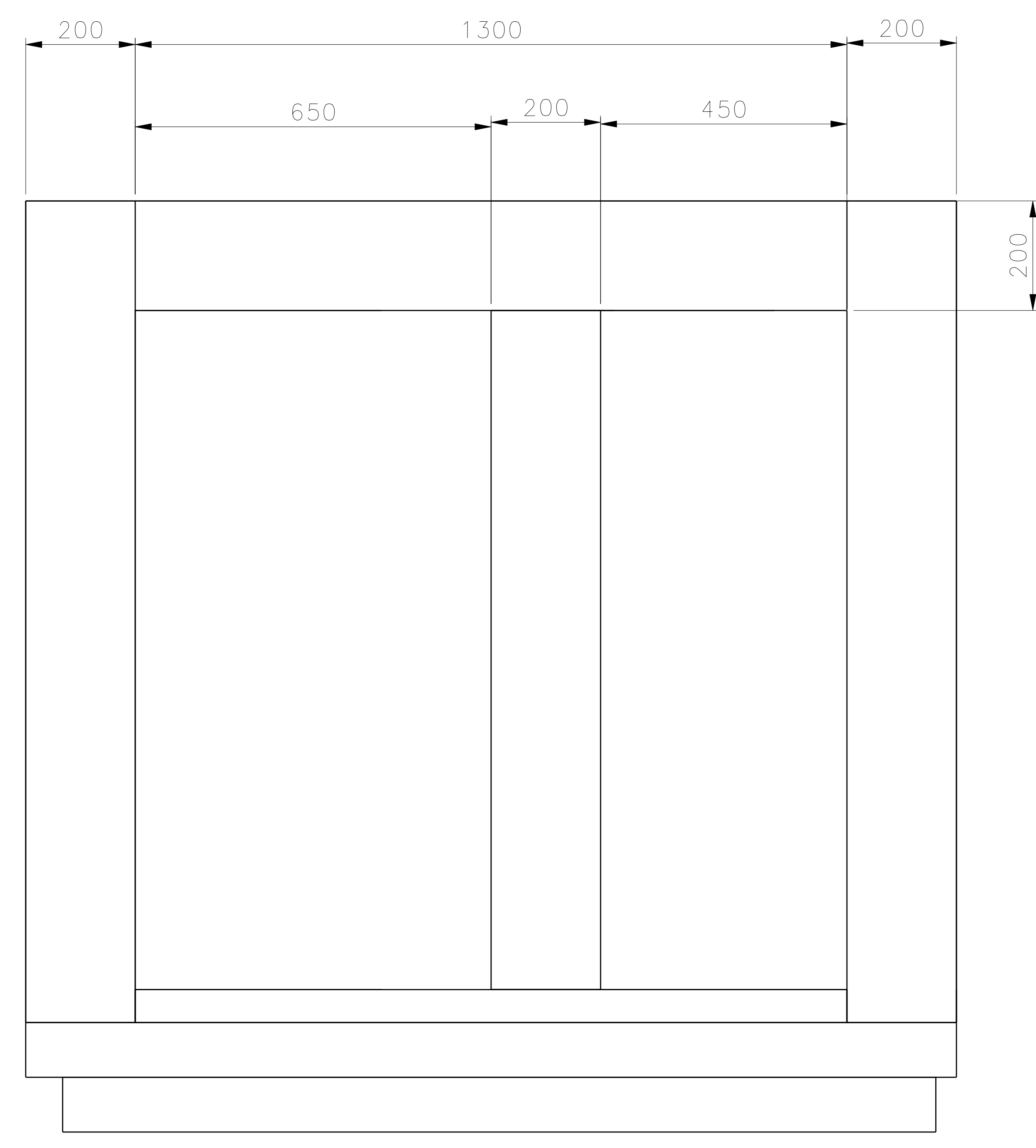
Right view Scale: 1:6
