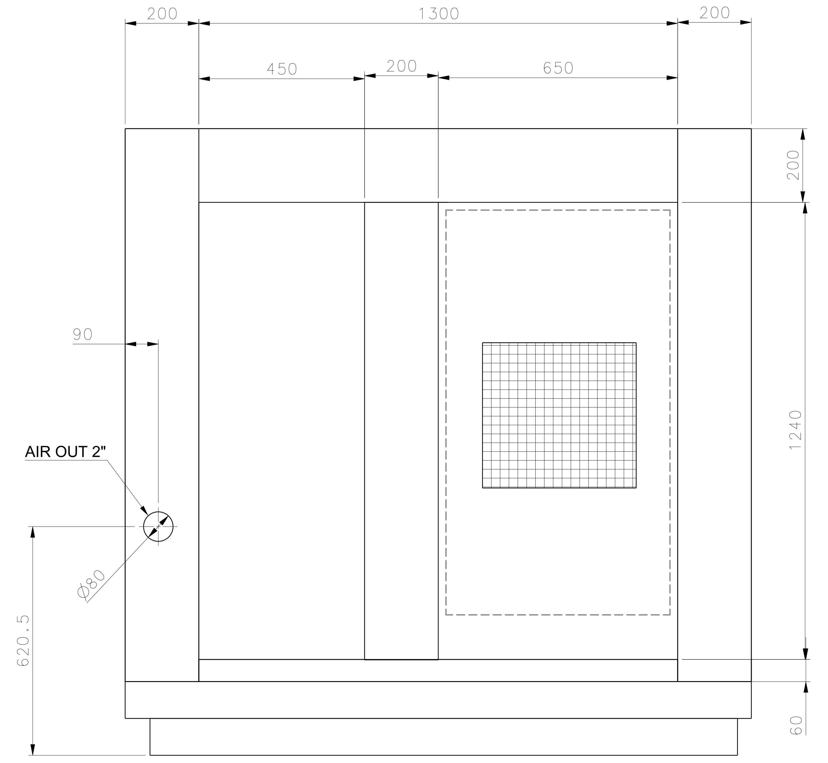
Left view Scale: 1:6
