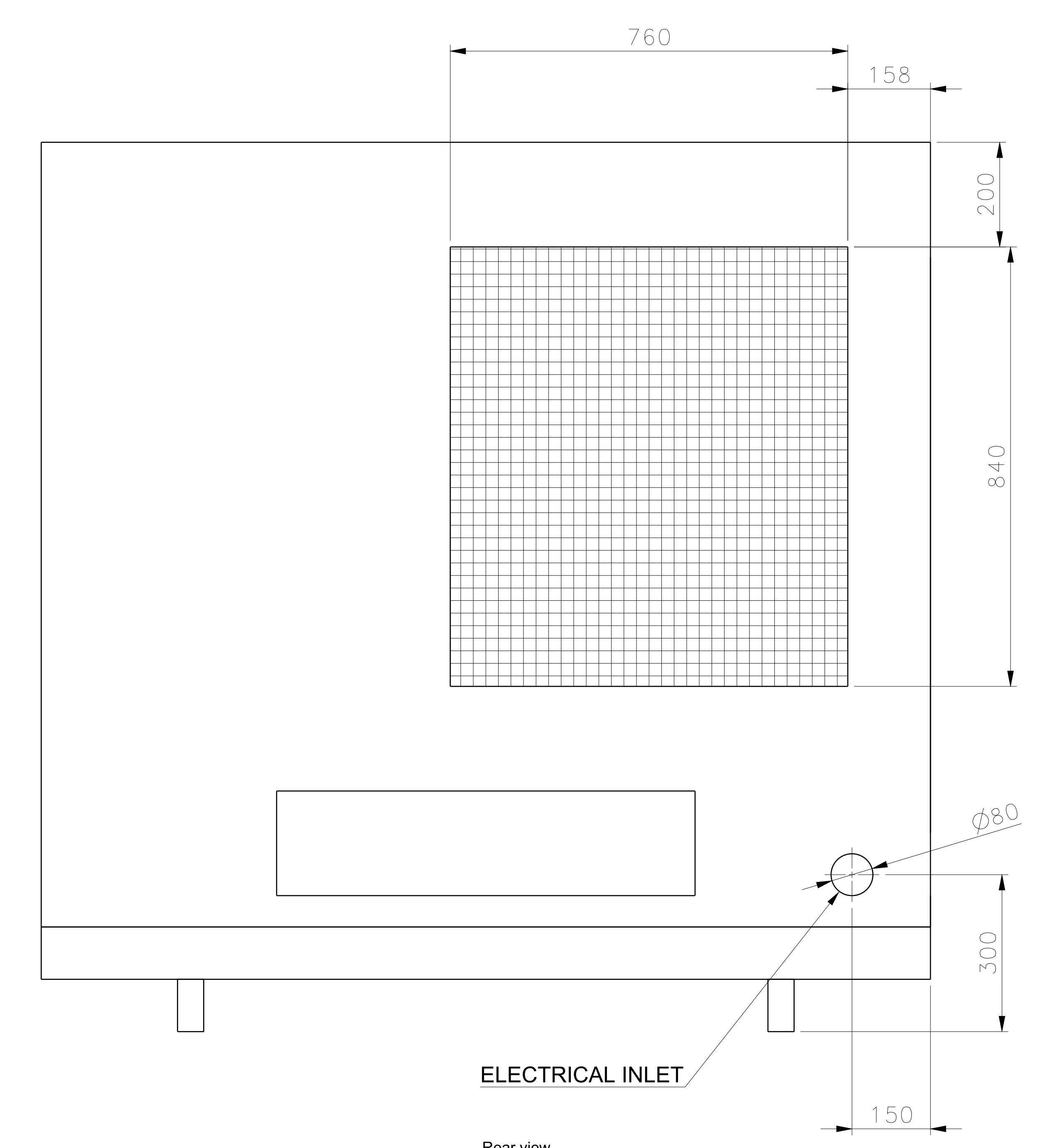
Rear view Scale: 1:6
