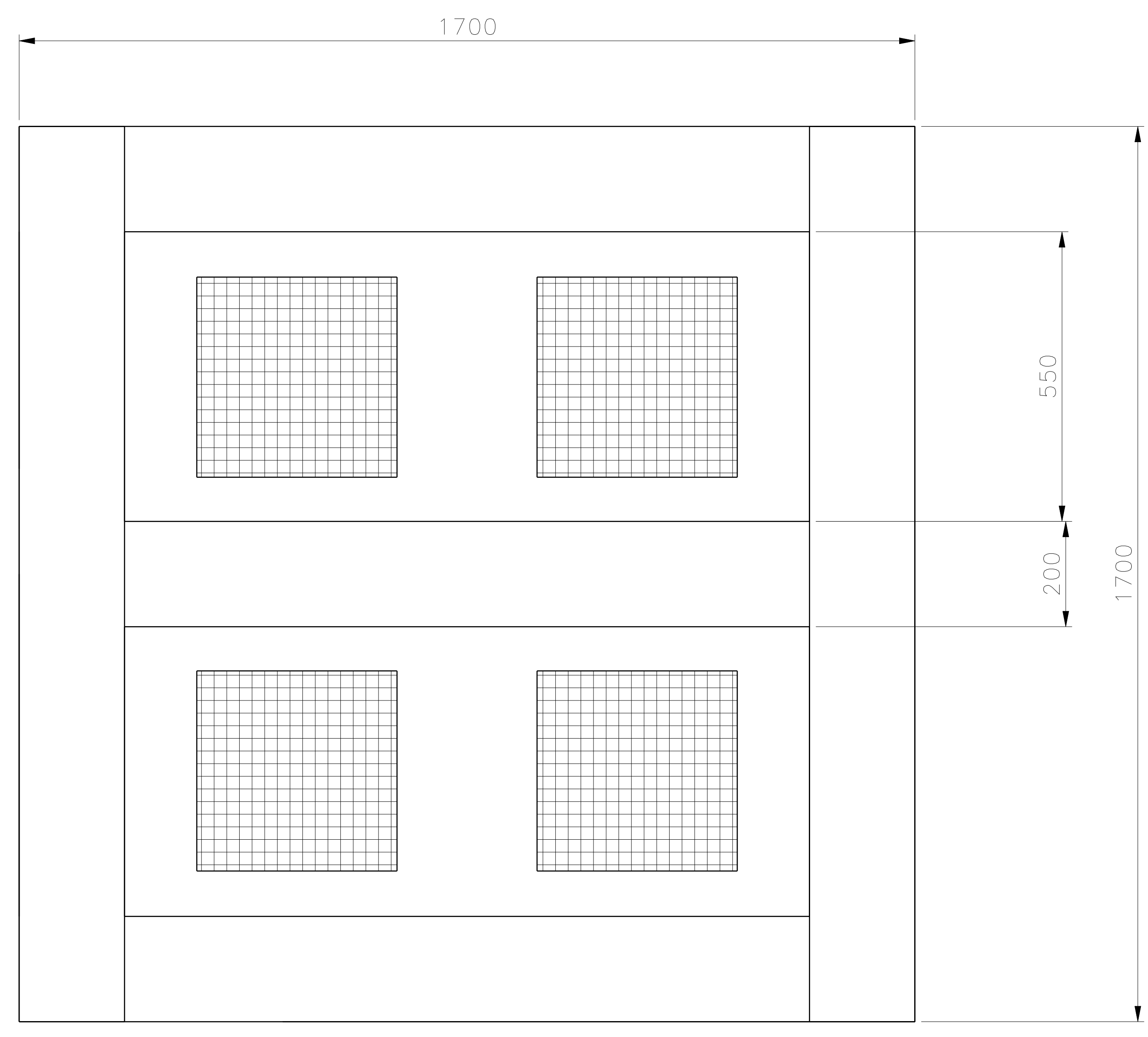
Top view Scale: 1:6
