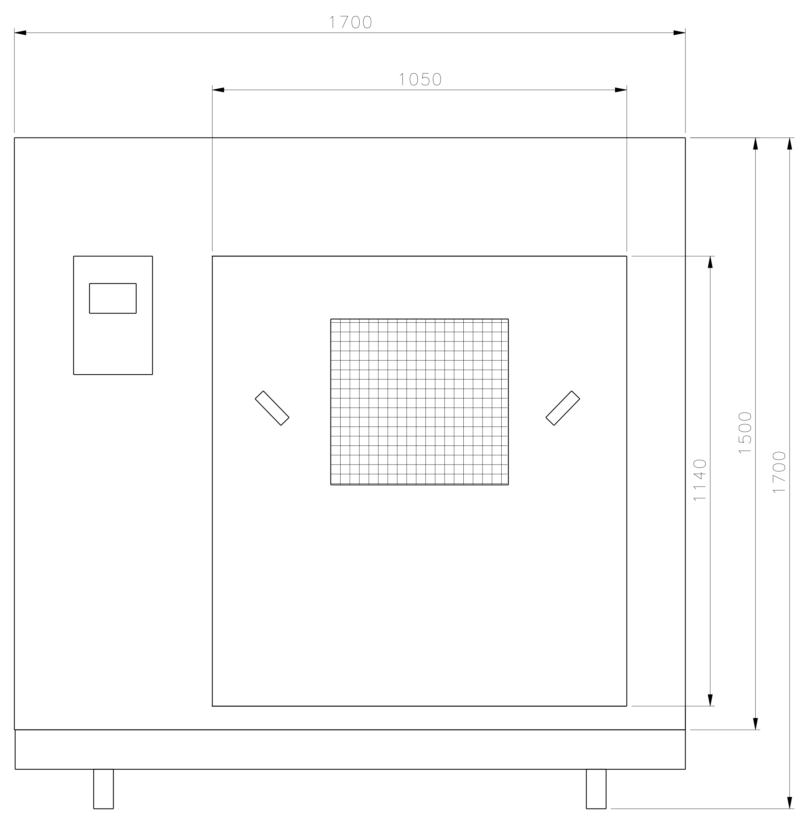
Front view Scale: 1:6
